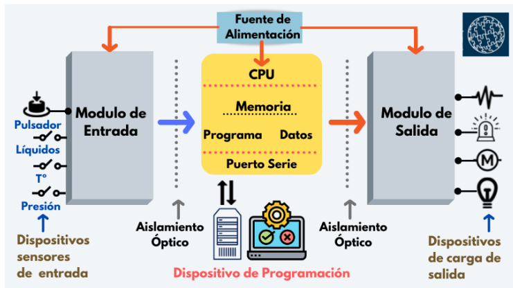
Figure: Componentes y funcionamiento de PLC [2].
